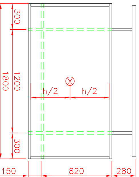
TYPRÄCKE 2 SKIVMITRL. / GLAS I RAM, MED UTSTICK, TÄCKT PLATTKANT.
