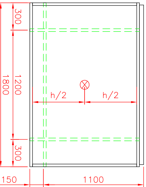
TYPRÄCKE 3 SKIVMITRL. / GLAS I RAM, MED UTSTICK, FULL HÖJD.
