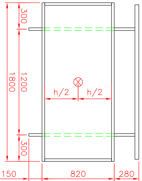
TYPRÄCKE 1 SKIVMITRL. / GLAS I RAM, MED UTSTICK.
